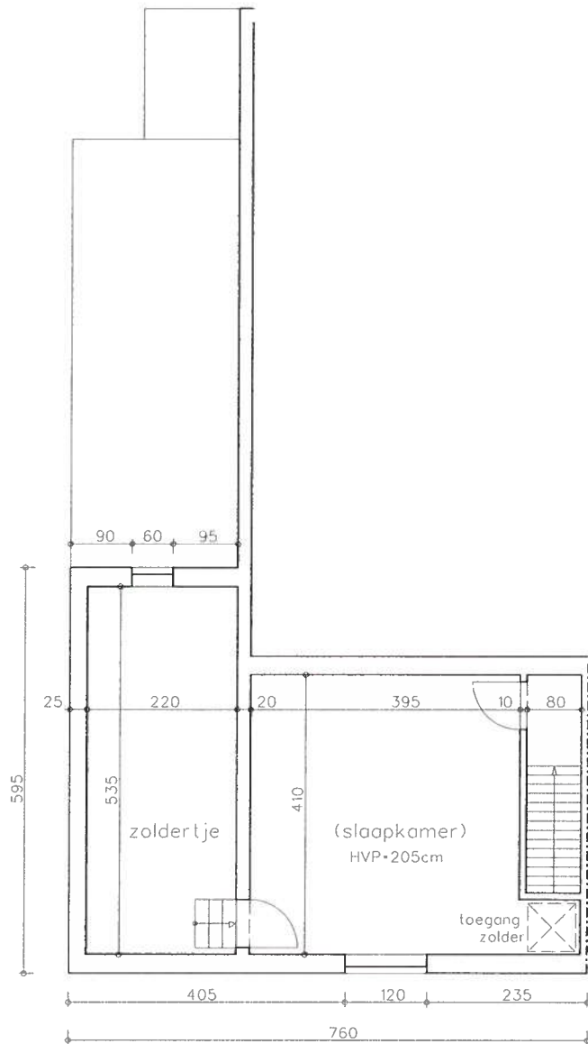
EERSTE VERDIEPING schaal 1/100 BESTAANDE TOESTAND
