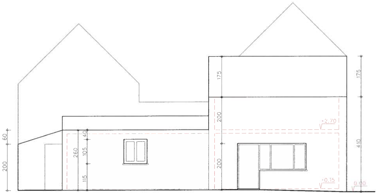
ZIJGEVEL schaal 1/100 BESTAANDE TOESTAND - ONGEWIJZIGD PLANNEN BRANDWEER
