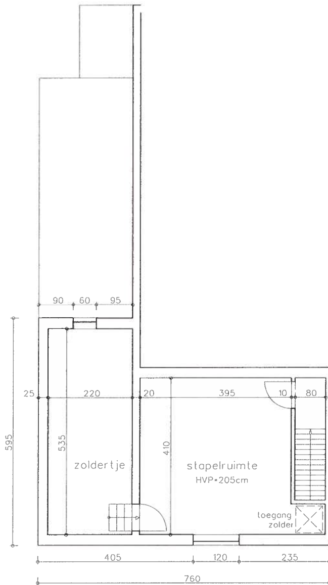
EERSTE VERDIEPING schaal 1/100 NIEUWE TOESTAND
