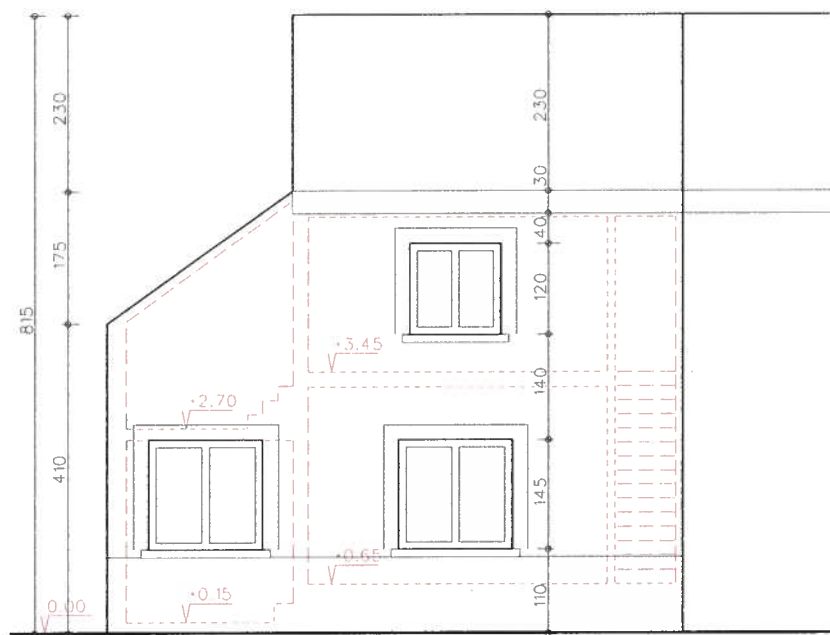
VOORGEVEL schaal 1/100 BESTAANDE TOESTAND - ONGEWIJZIGD PLANNEN BRANDWEER
